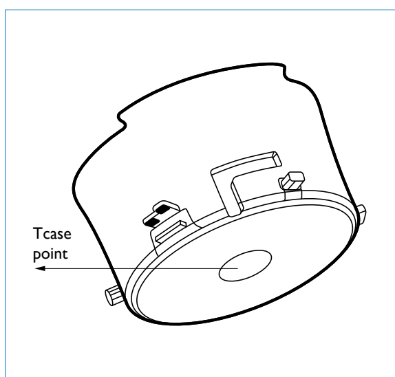
T_{case} point
